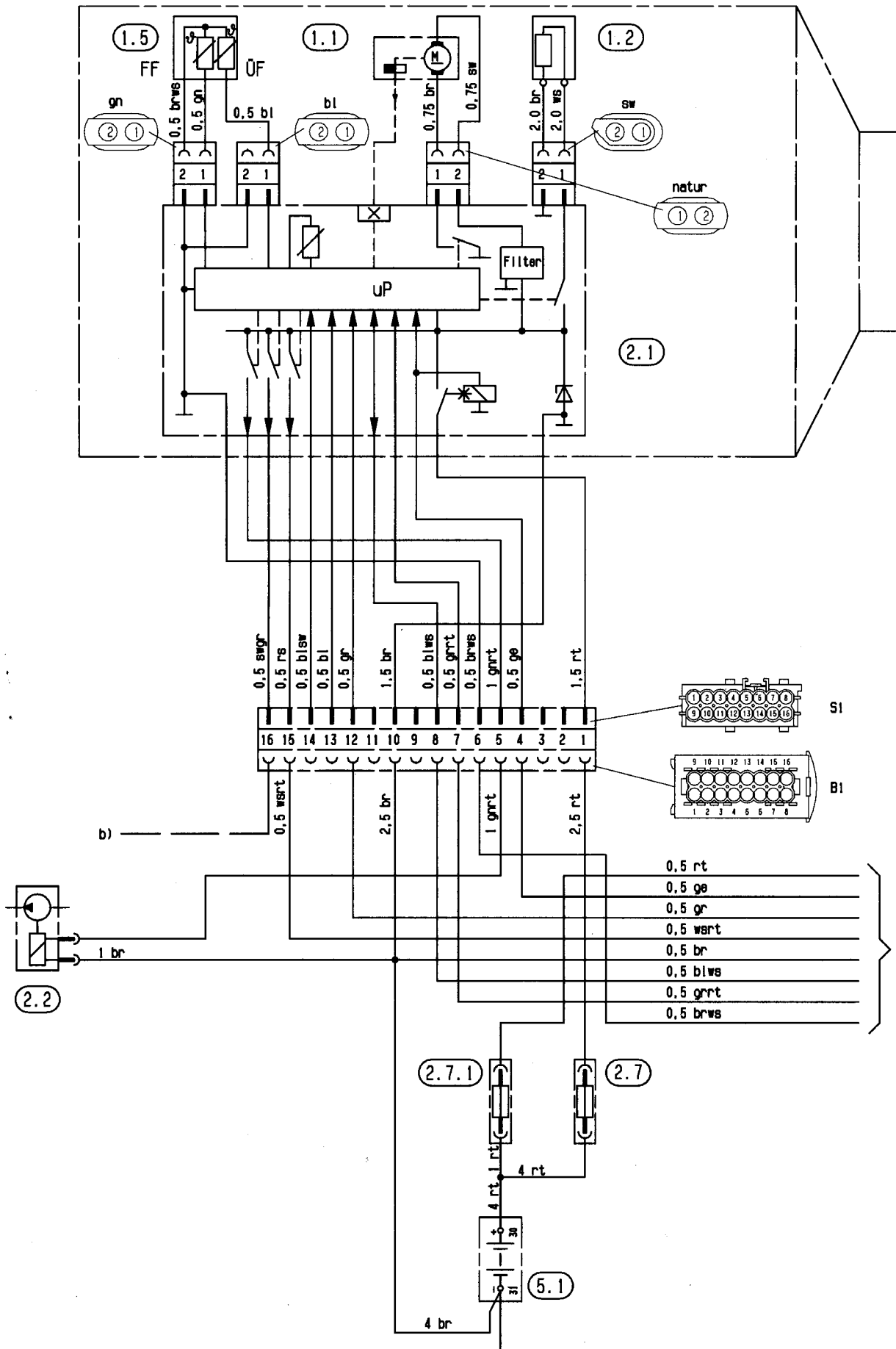
SCHEMA ELECTRIQUEAIRTRONIC D2 / AIRTRONIC D4 (OPTION)
